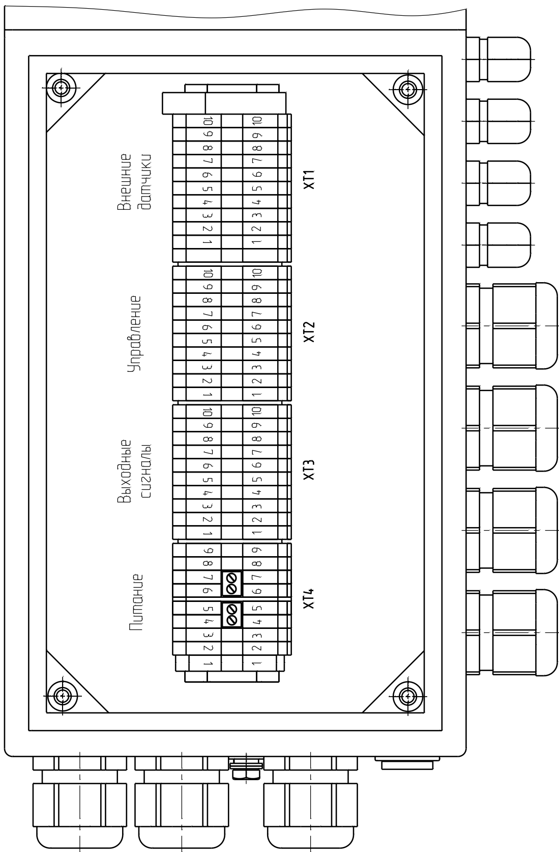
Рис.Ж.3 Расположение клемм в коммутационном блоке горелки
