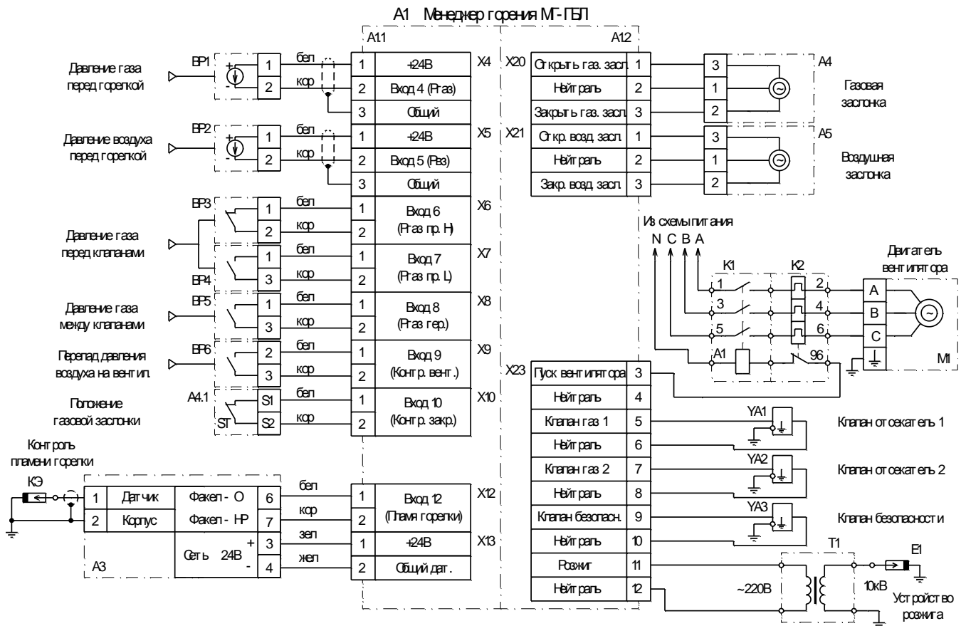
Вариант подключения устройств контроля пламени Г-ПСЭ-1
