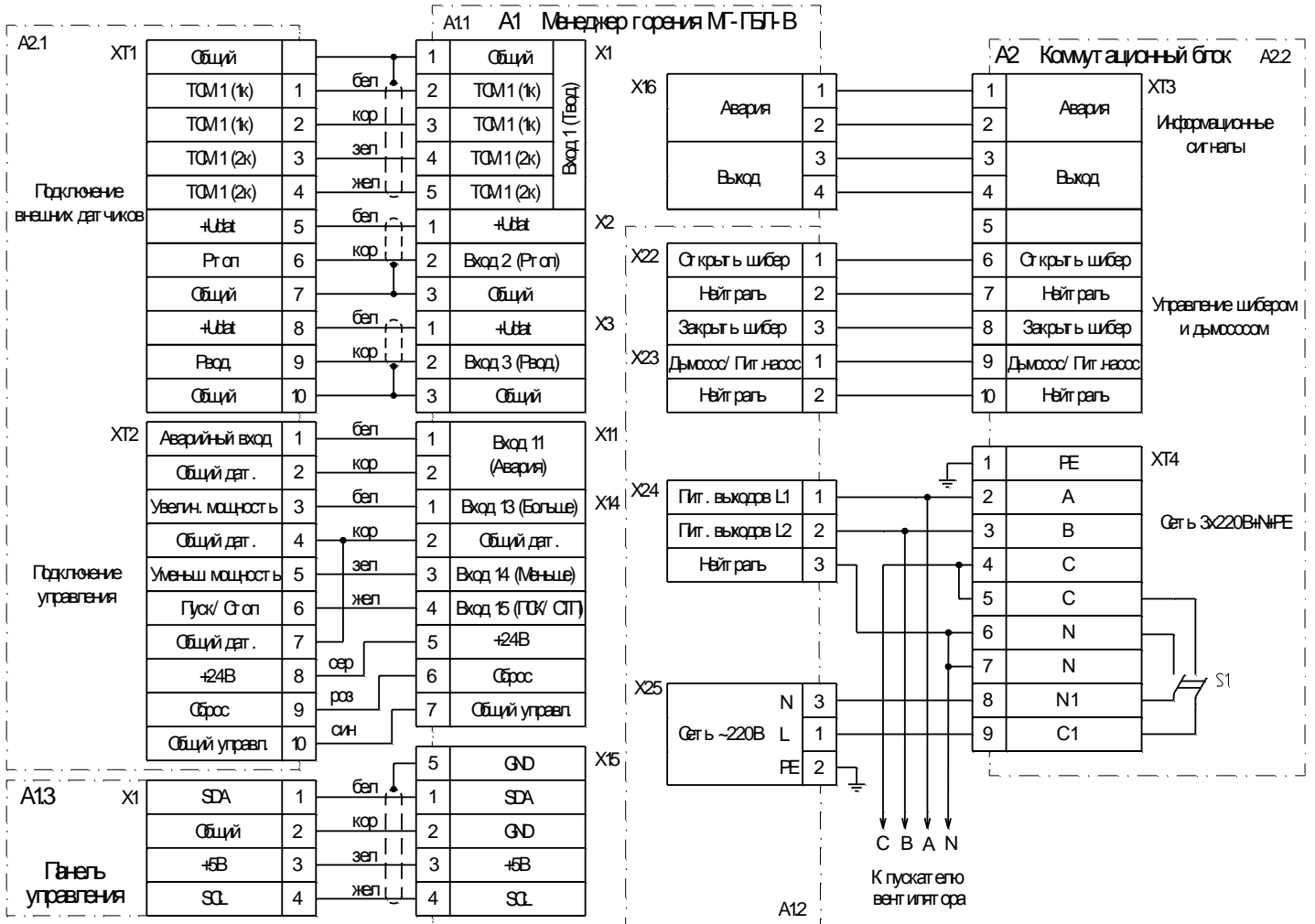
Подключение внешних датчиков для варианта М-ГБТ-П с токовым входом регулятора производительности
