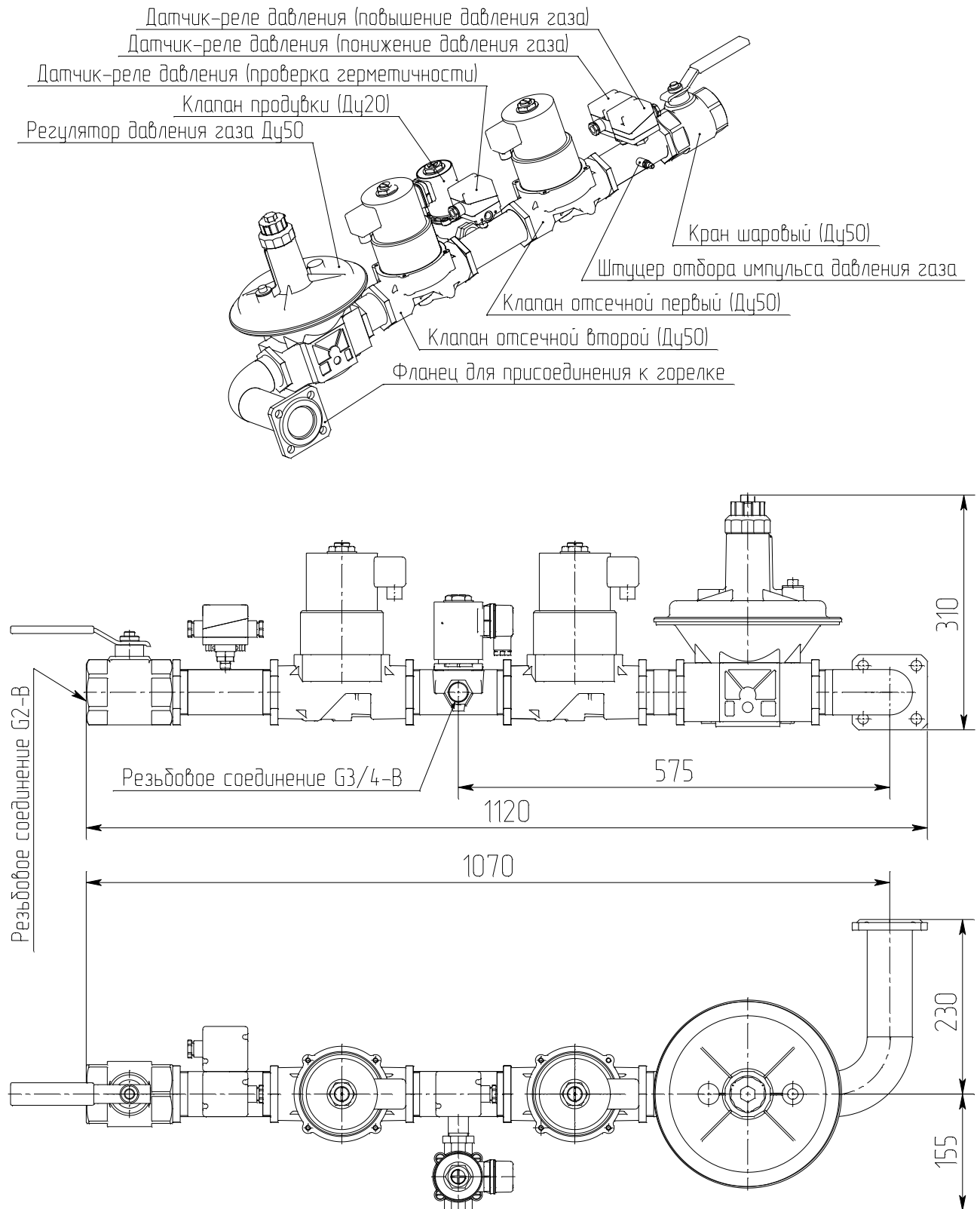
Рисунок Б.1. Группа арматурная Ca6.617.063 (Ca6.617.063-06)
